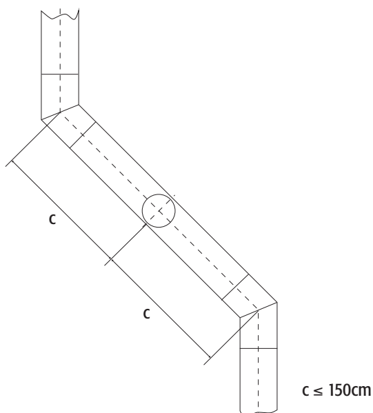
Bild 3 – Abstand bei Reinigungsöffnung in einer Etage
